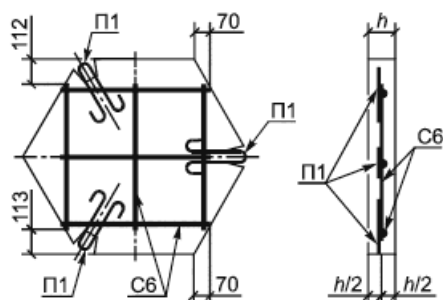
Рисунок Б.4 - Армирование тротуарной плиты 3Ш
