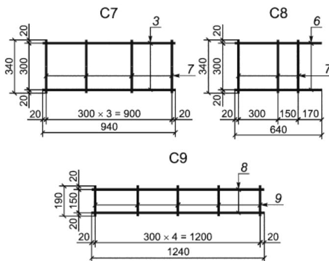
Рисунок Б.11 - Арматурные сетки С7, С8, С9
