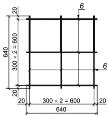
Рисунок Б.10 - Арматурная сетка С6
