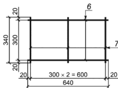
Рисунок Б.12 - Арматурная сетка С10
